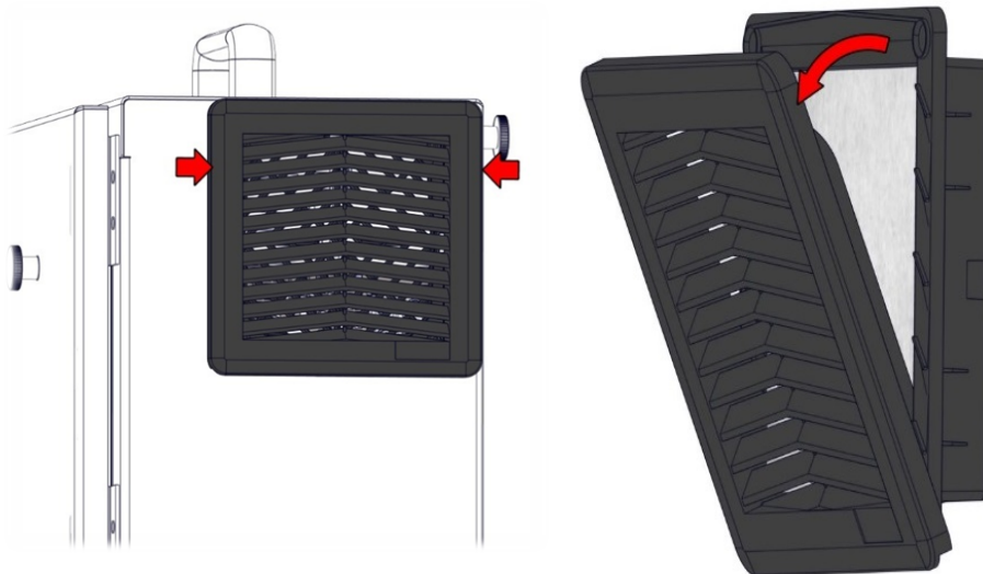
3.7. ábra Cserélje ki a vezérlődoboz szűrőit.
