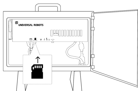
Vezérlődoboz
