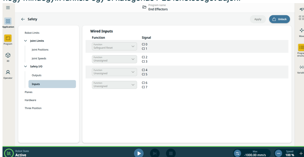
Ábra 1.4 : A PolyScope X képernyője a megjelenített bemeneti jelekkel.
