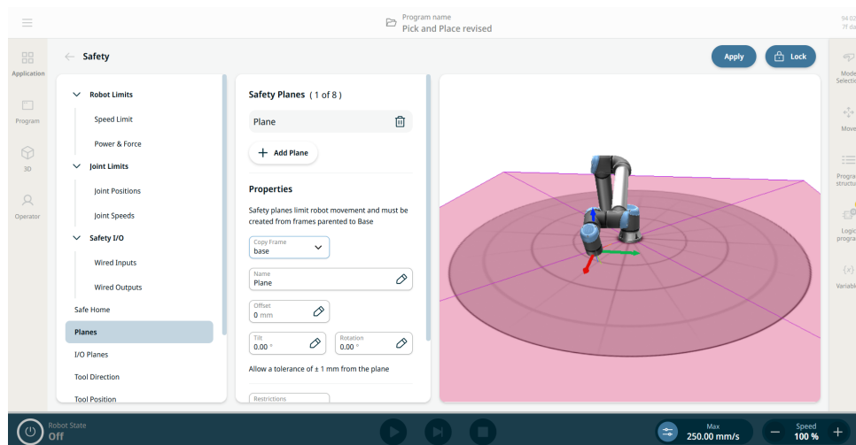
Ábra 1.5: PolyScope X képernyő megjelenített biztonsági síkokkal.
